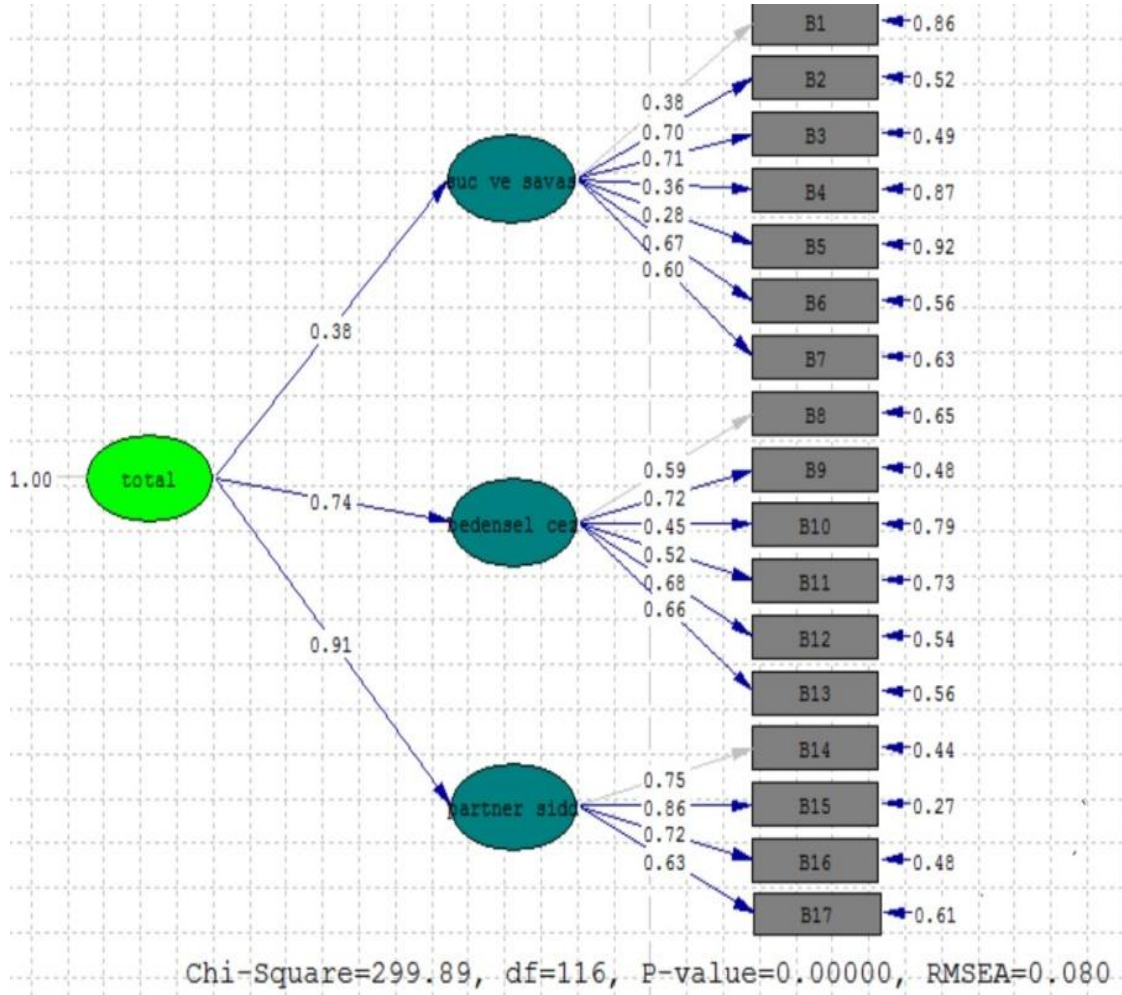
Şekil 2. Şiddete Yönelik Tutum Ölçeğine İlişkin İkinci Düzey Doğrulayıcı Faktör Analizi
