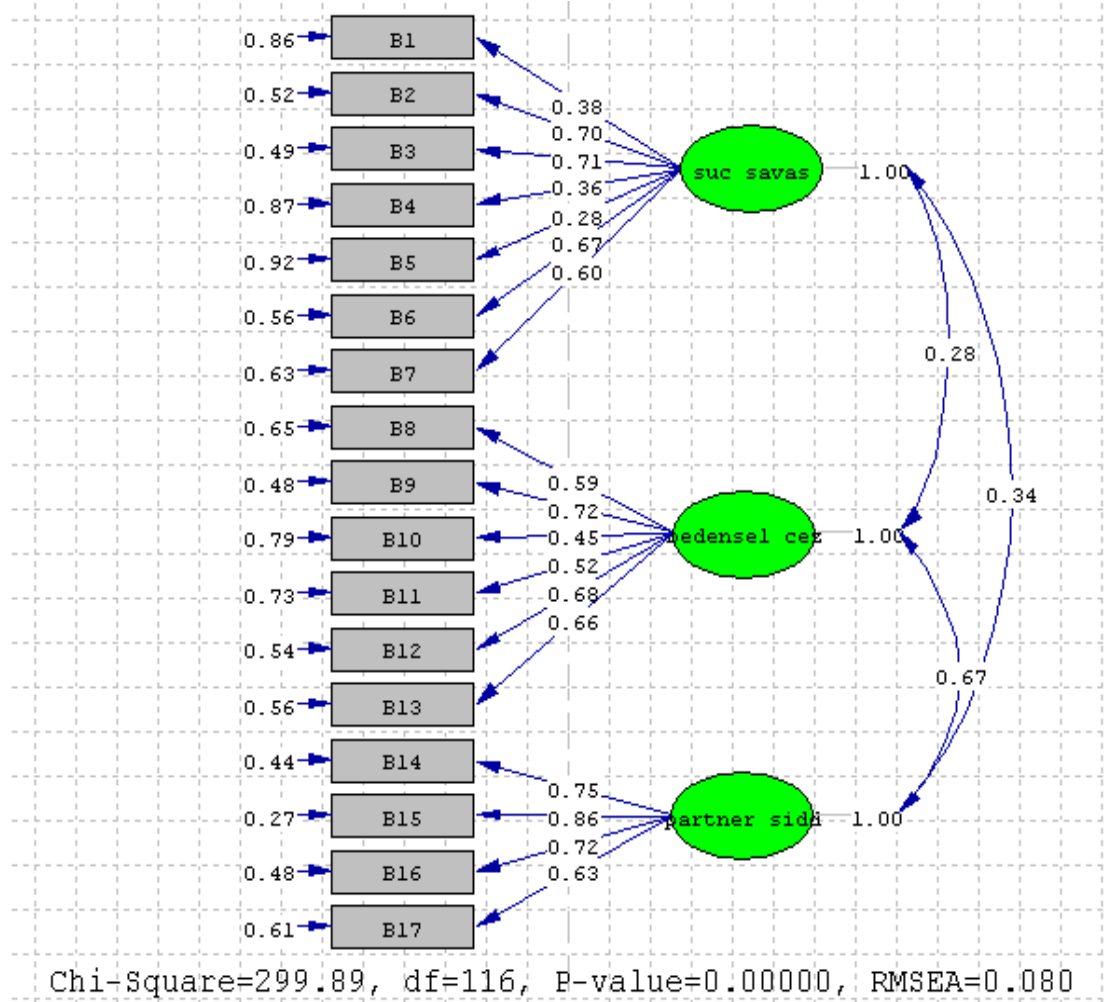
Şekil 1. Şiddete Yönelik Tutum Ölçeğine İlişkin Birinci Düzey Doğrulayıcı Faktör Analizi
